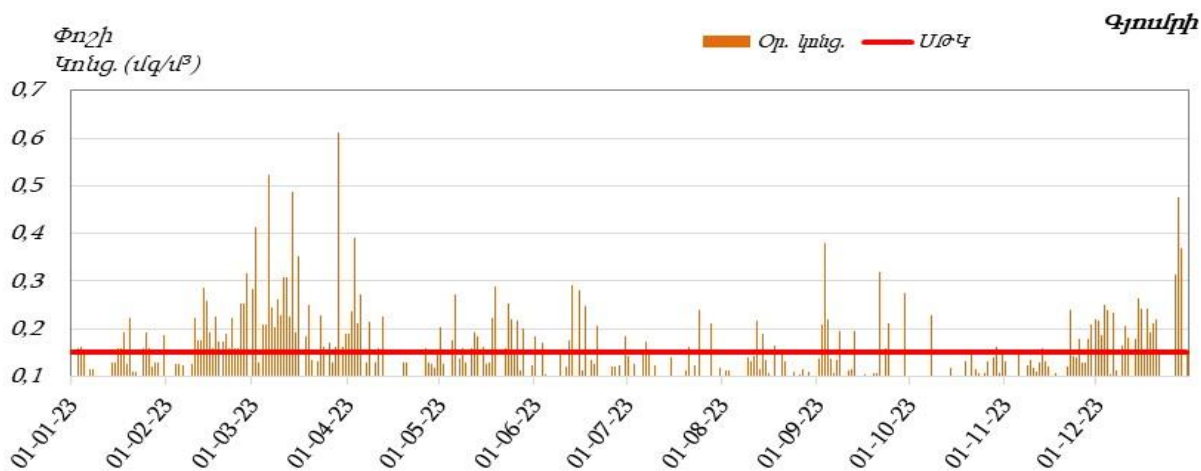
Գծապատկեր 12. Գյուճրի քաղաքի մթնոլորտային օդում փոշու օրական կոնցենտրացիայի փոփոխությունները 2023 թ.
