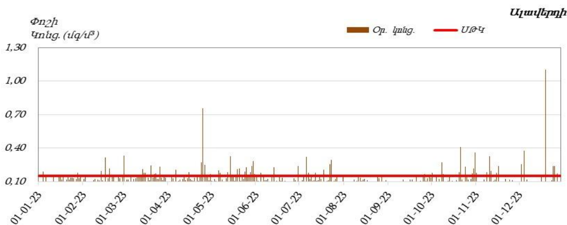
Գծապատկեր 20. Ալավերդի քաղաքի մթնոլորտային օդում փոշու օրական կոնցենտրացիայի փոփոխությունները 2023 թ.
