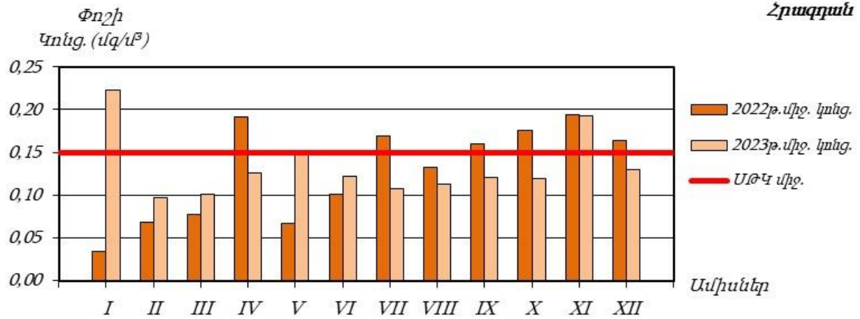
Գծապատկեր 25. Հրագրան քաղաքի մթնոլորտային օդում փոշու միջին ամսական կոնցենտրացիաների փոփոխությունները
