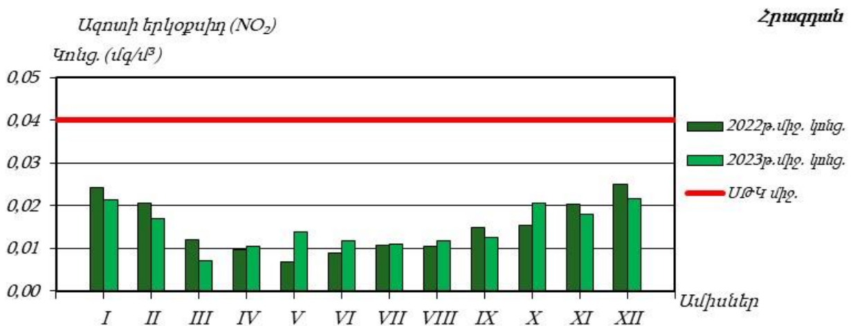
Գծապատկեր 27. Հրագրան քաղաքի մթնոլորտային օդում ազոտի երկօքսիդի միջին ամսական կոնցենտրացիաների փոփոխությունները
