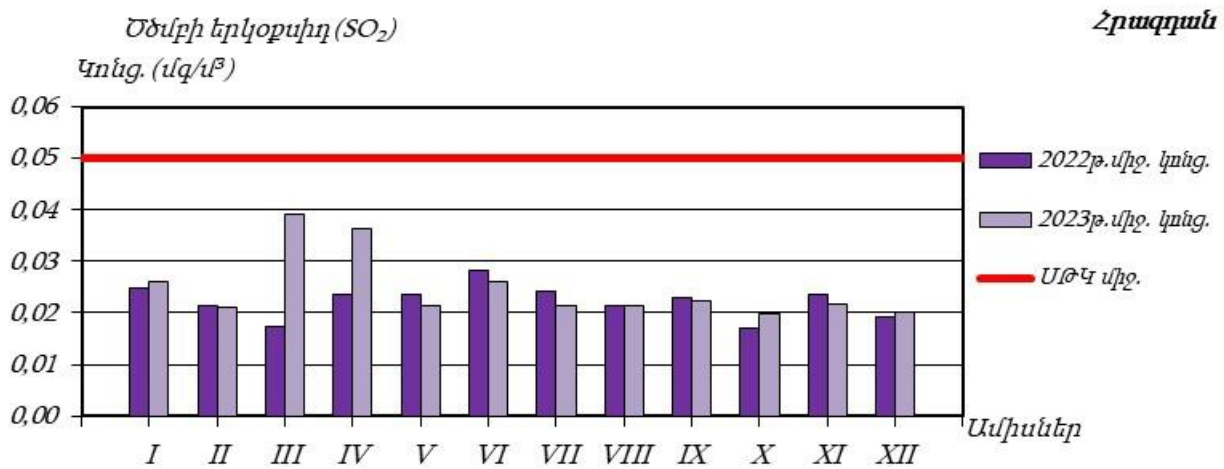
Գծապատկեր 26. Հրագրան քաղաքի մթնոլորտային օդում ծծմբի երկօքսիդի միջին ամսական կոնցենտրացիաների փոփոխությունները
